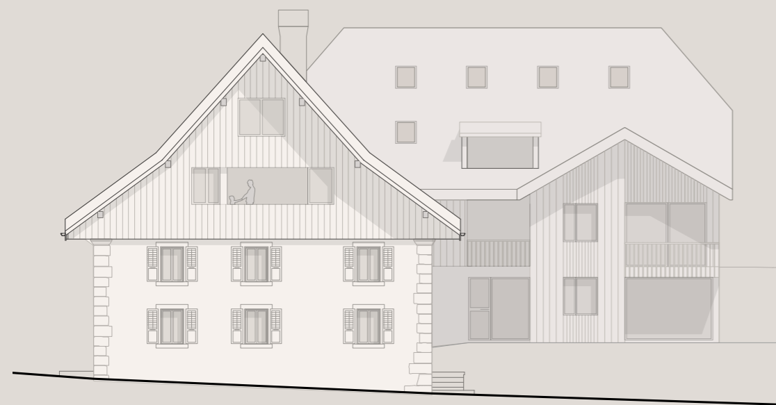
façades ouest
